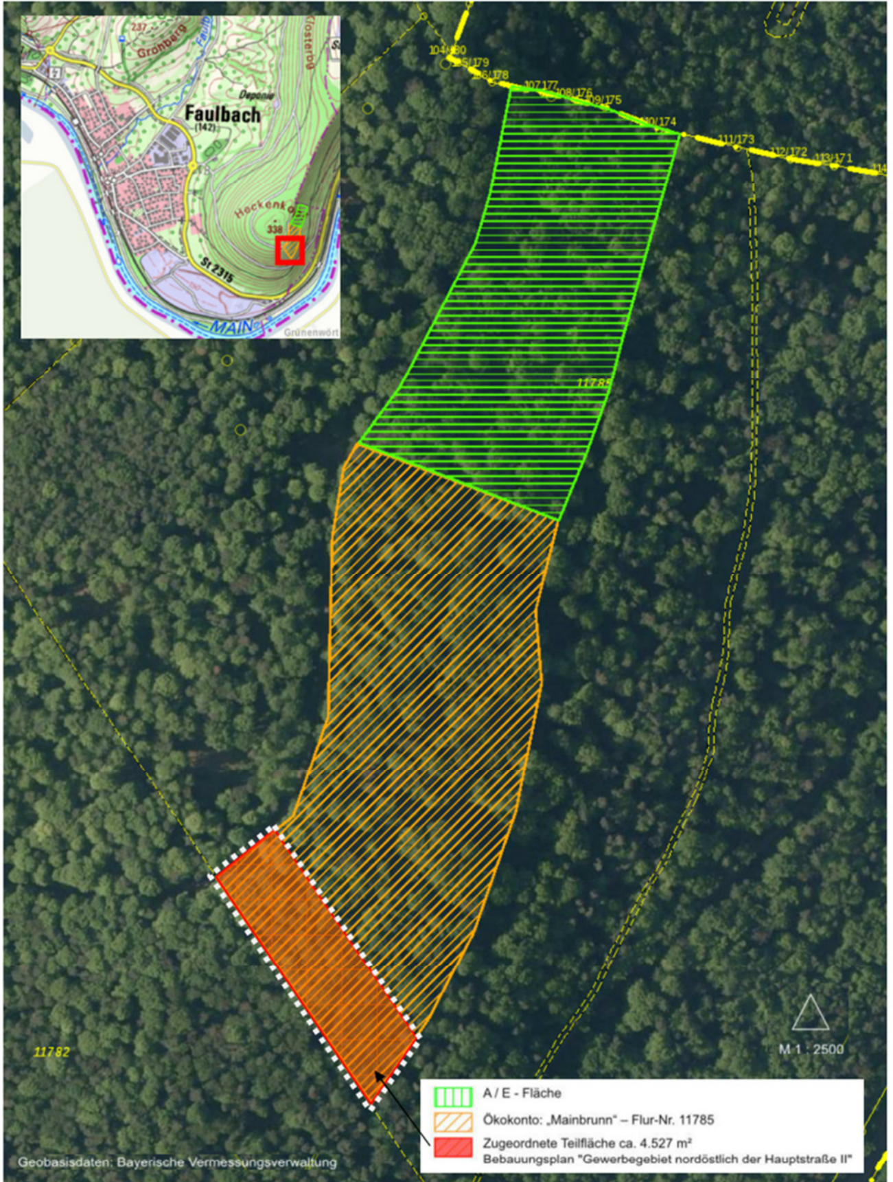
Gemeinde Faulbach: Bebauungsplan Gewerbegebiet nordöstlich Faulbach Ausgleichsfläche „Mainbrunn“ Fl.Nr. 11785 (Gmkg. Faulbach) – Teilfläche 4.527 m 2 Lageplan M. = 1:2.500
